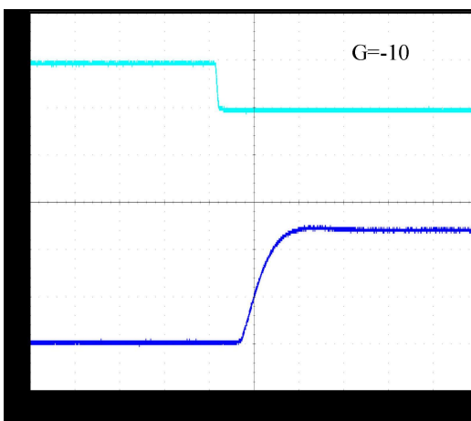
图 7 负过载恢复
