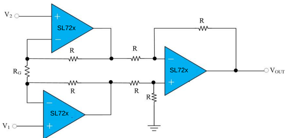
图 17 仪表放大器
