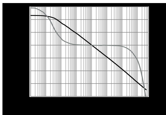
图 12 开环增益和相位与频率的关系
