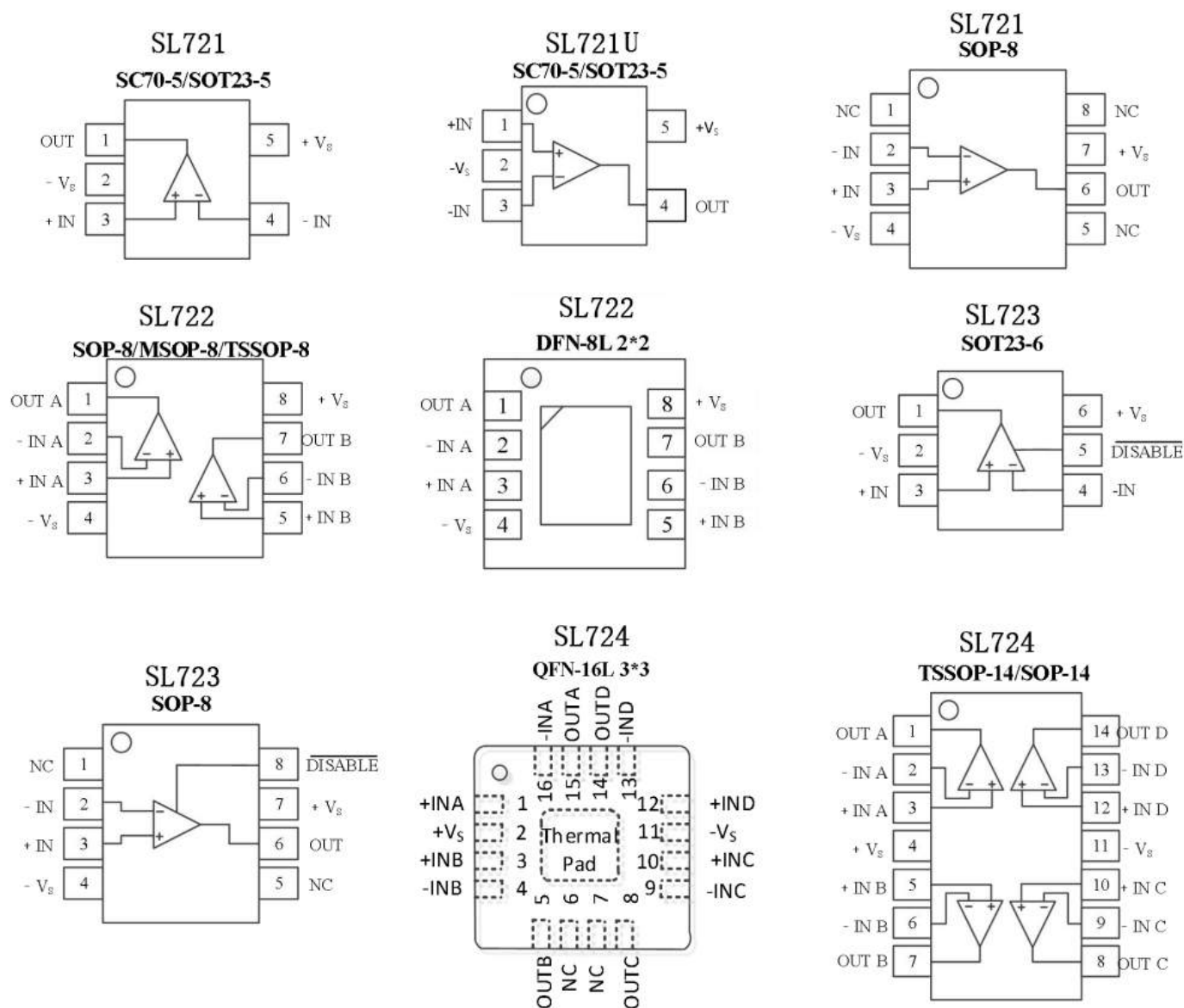
图 1 管脚分布
